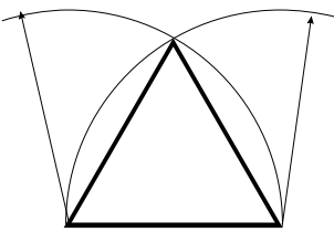
Triángulo equilátero
