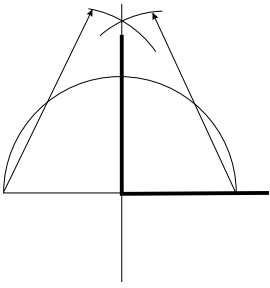
Ángulo de 90°
