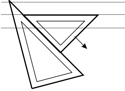
Verticales con escuadra y cartabón
