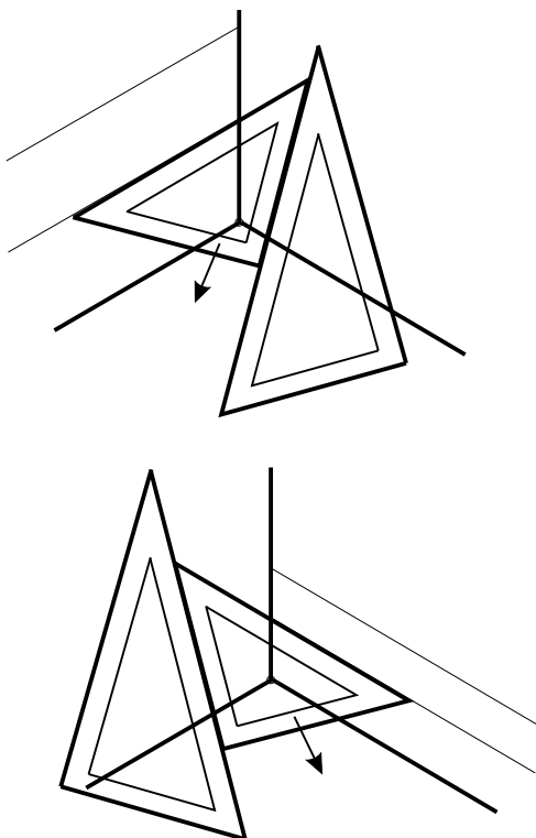
Paralelas a los ejes axonométricos
