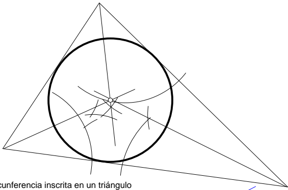
Circunferencia inscrita en un triángulo
