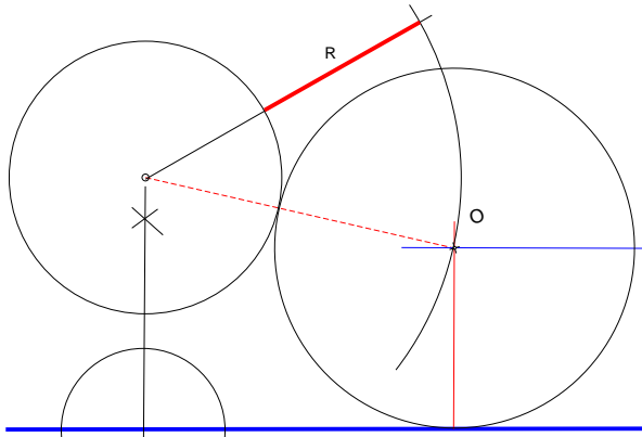
Circunferencia de radio R=20 tangente a otra y a una recta
