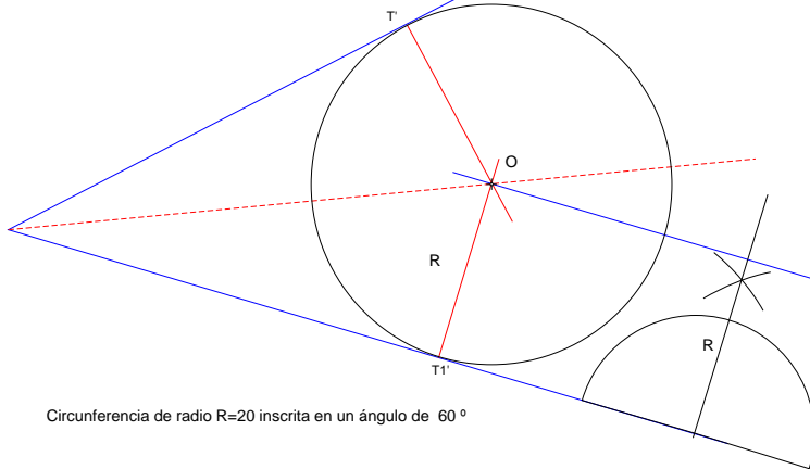
Circunferencia de radio R=20 inscrita en un ángulo de 60^\circ
