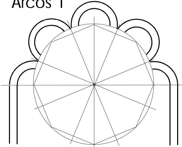
Arco festoneado de 5 centros
